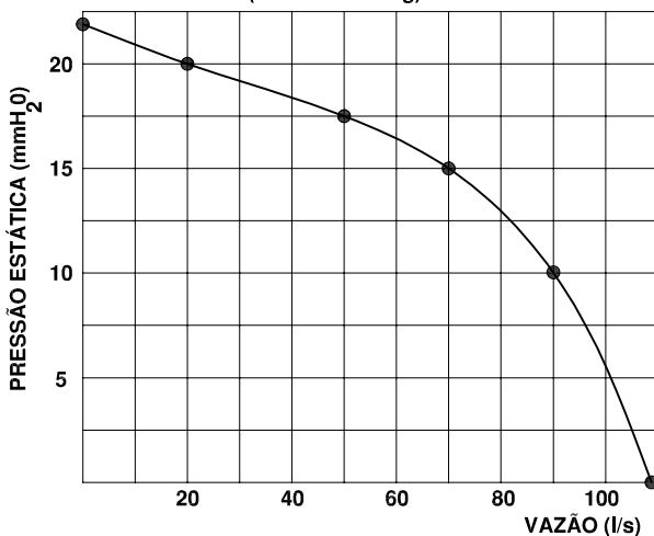
CURVA CARACTERÍSTICA (20°C/760 mmHg)
